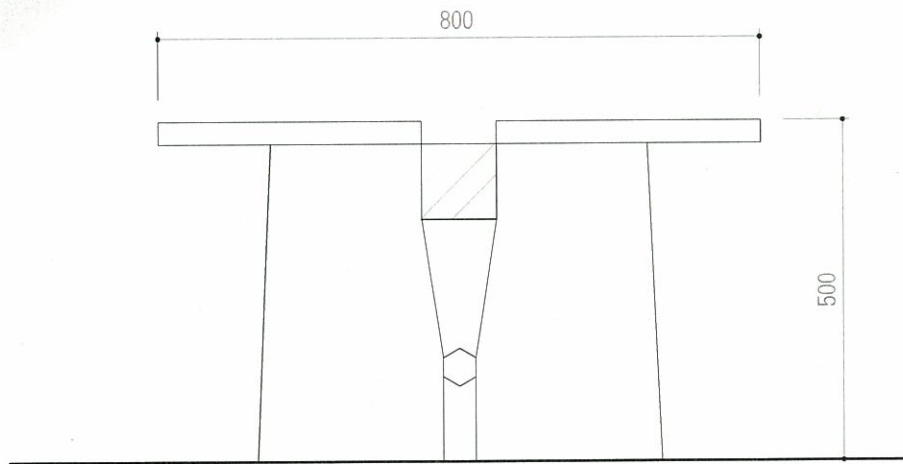
短手立面図 1/10
