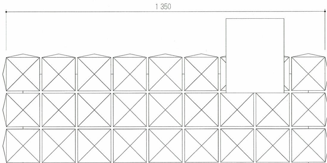
長手立面図 1/10
